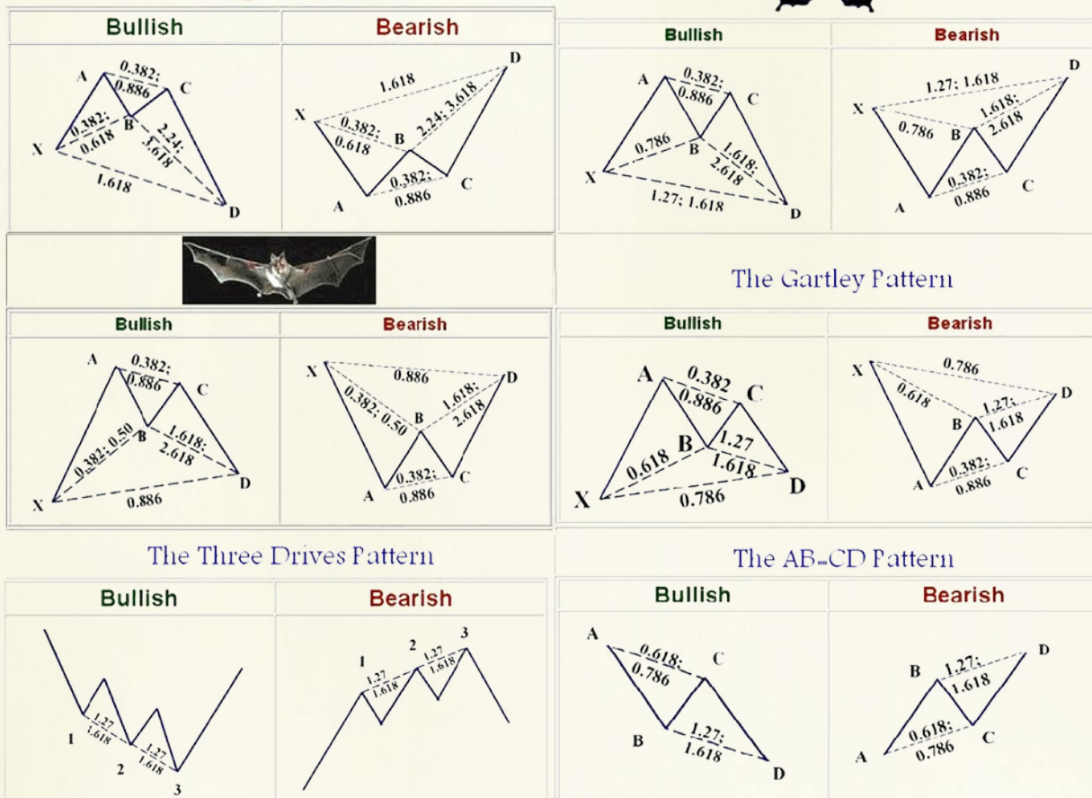
Рис. 1. Паттерны Гартли
